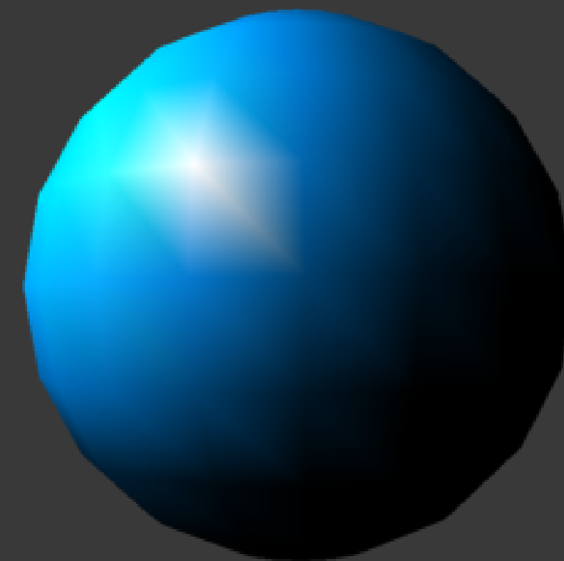
GOURAUD SHADING
